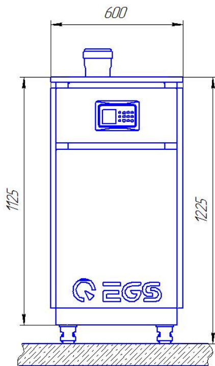
Общий вид спереди EGS ALUM-F 1.80/120
