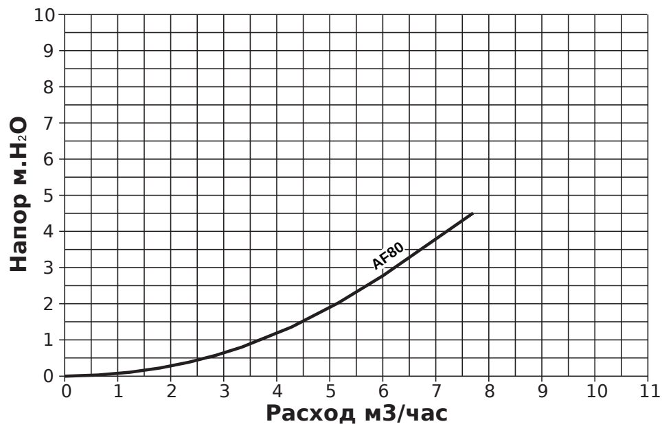
Диаграмма потери нагрузки котла EGS ALUM-F1.80
