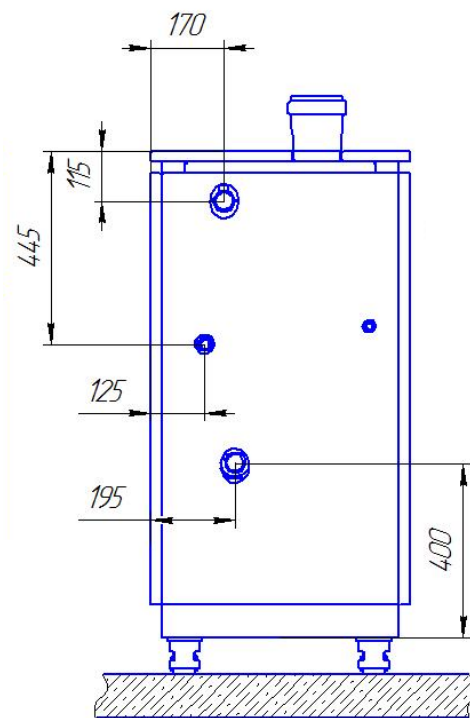
Общий вид спереди EGS ALUM-F 1.80/120
