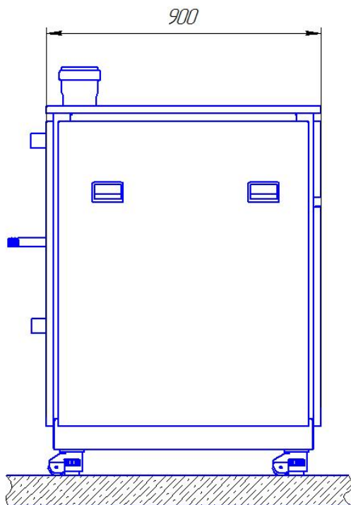
Общий вид сбоку EGS ALUM-F 1.80/120
