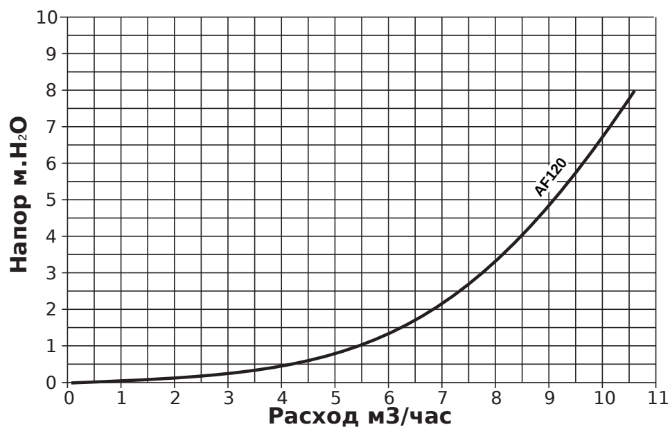
Диаграмма потери нагрузки котла EGS ALUM-F1.120
